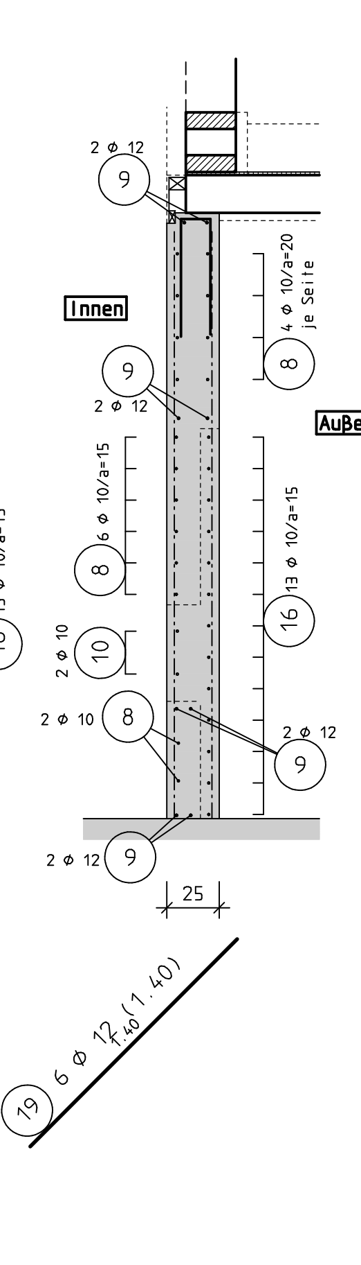
Schnitt 2-2
