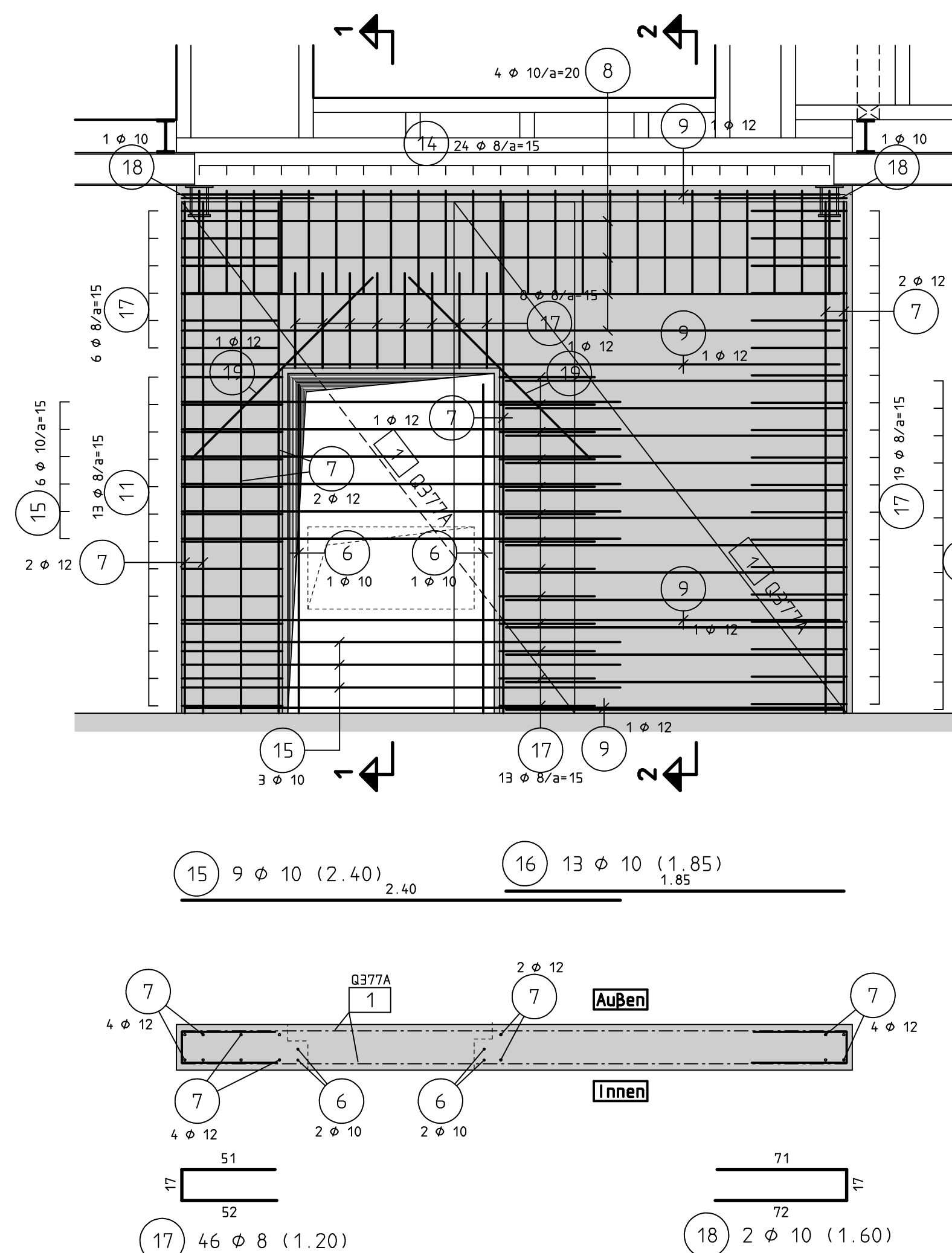
Bewehrung Außen
