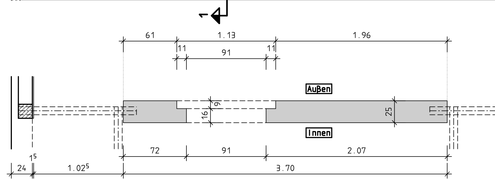
Bewehrung Innen
