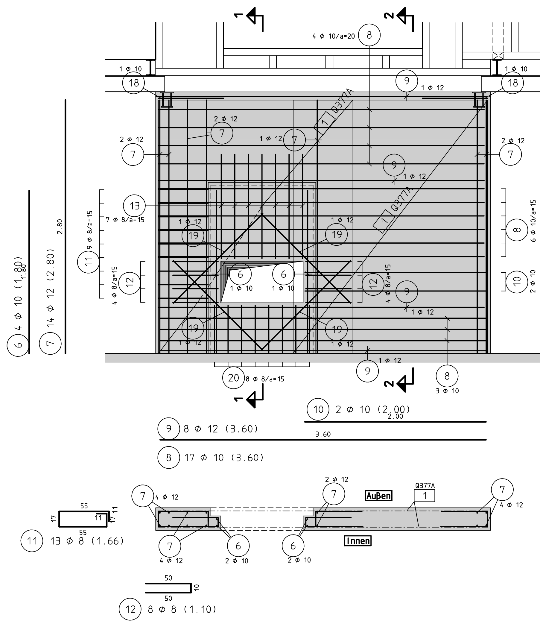
Bewehrung Innen
