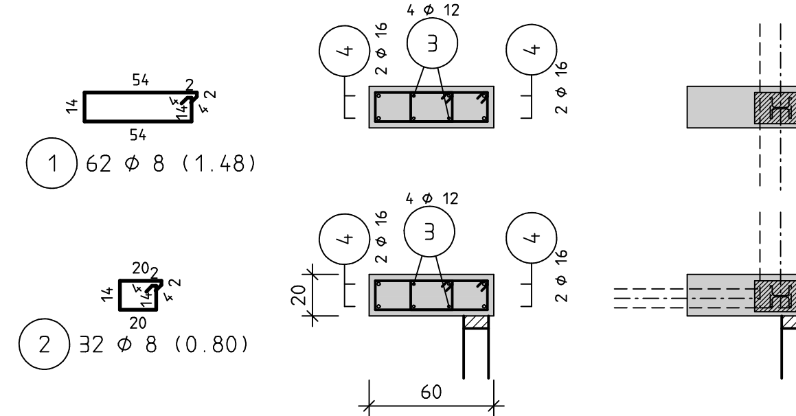
Bewehrung Außen
