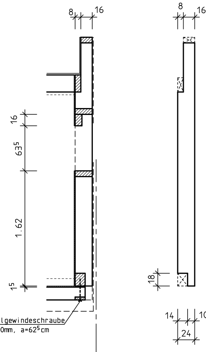
Schnitt 13.1
