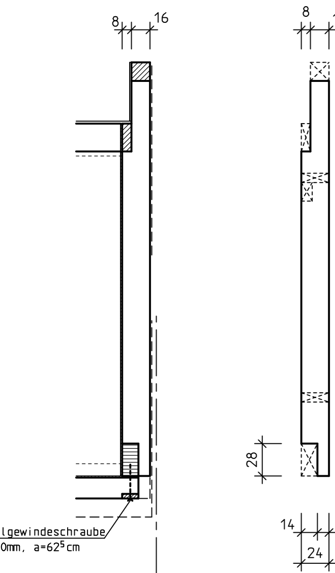
Schnitt 14.1
