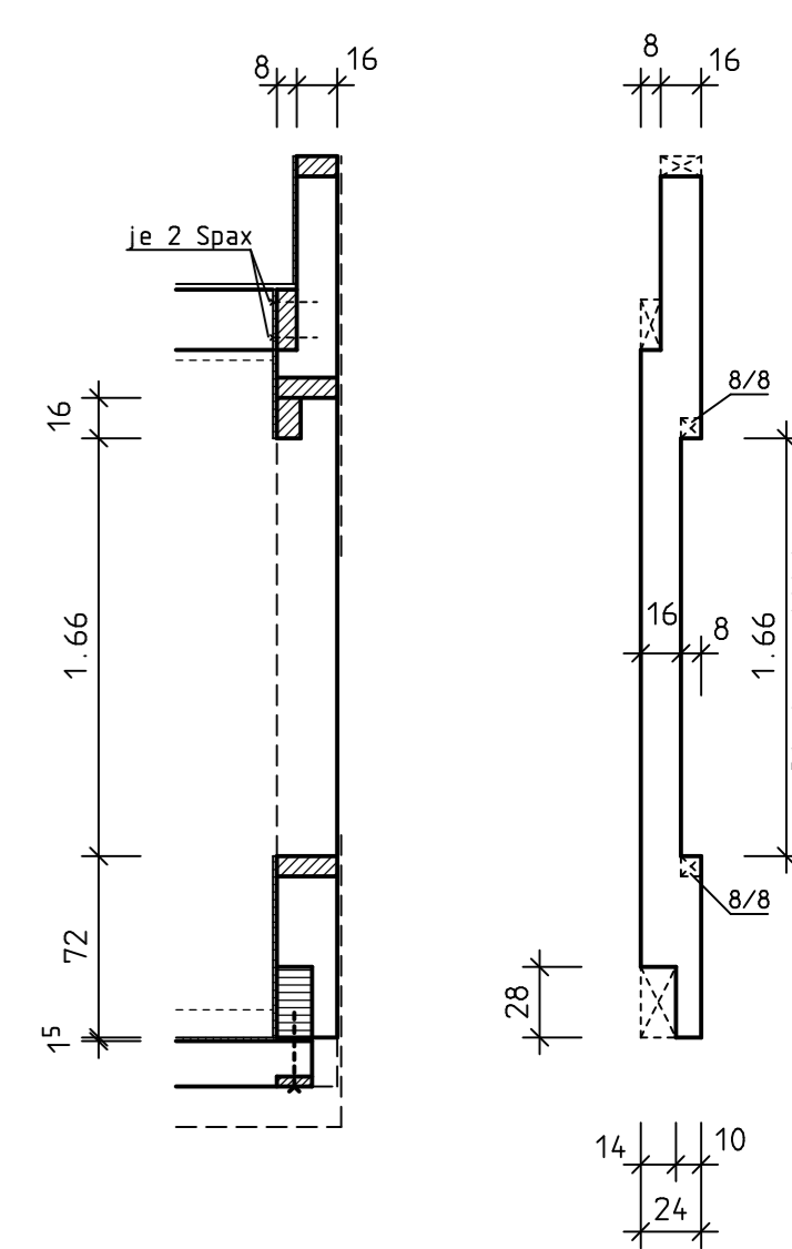
Schnitt 14.2
