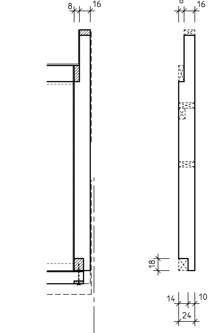
Schnitt 13.2
