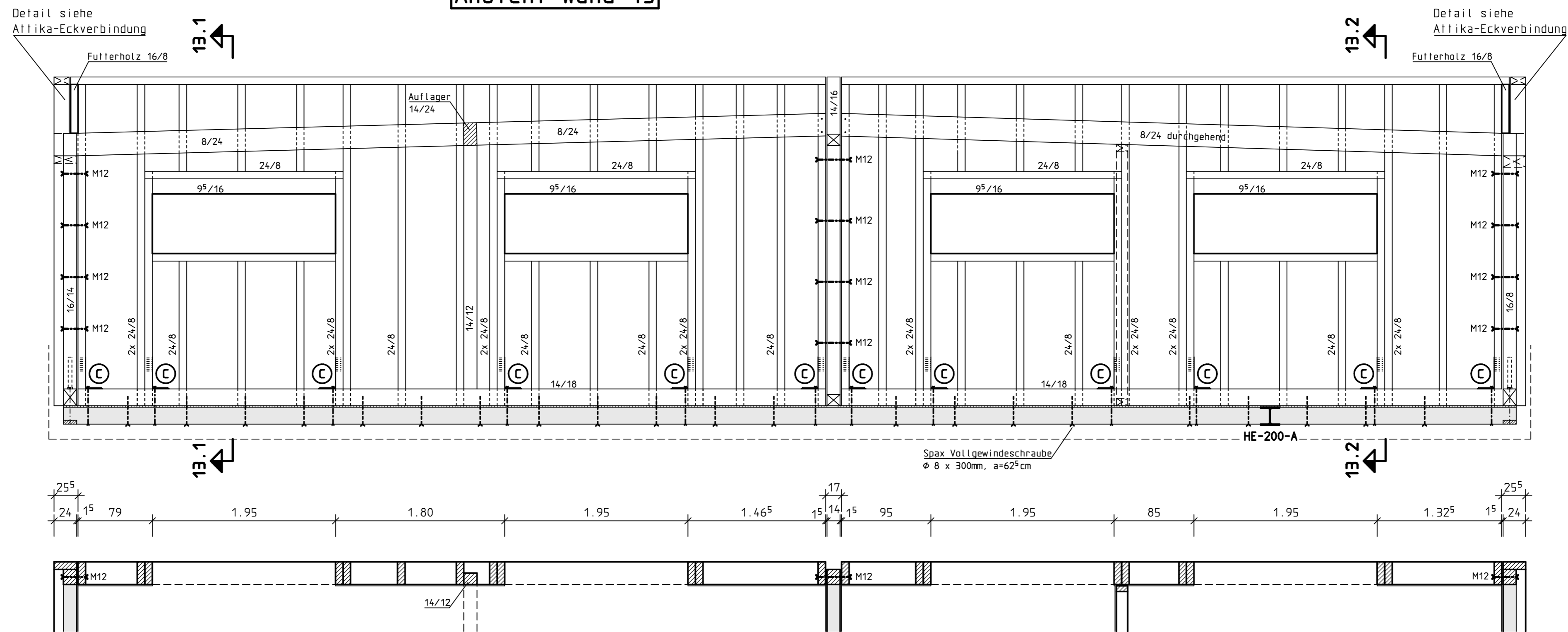
Ansicht Wand 13
